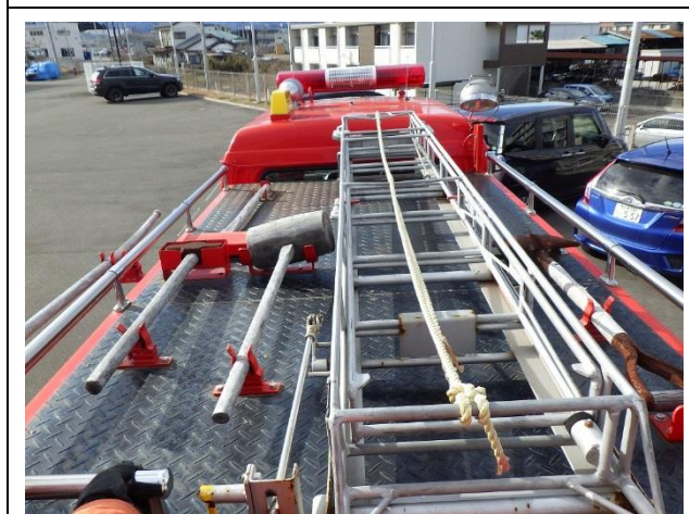
車体上部 (二連梯子、掛矢、斧、剣先スコップ)
